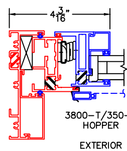
9 BLOCK JAMB
