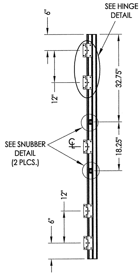
HINGE JAMB
