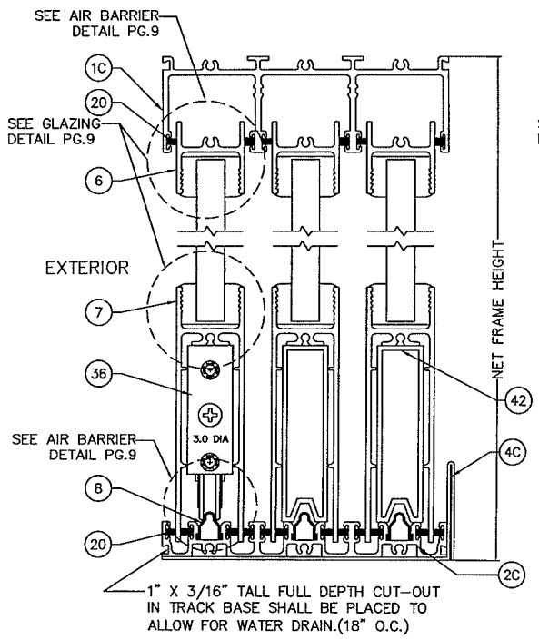
A1 SECTION 7 SCALE: 1/2 FULL
