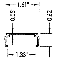
15 JAMB CHANNEL FILLER
