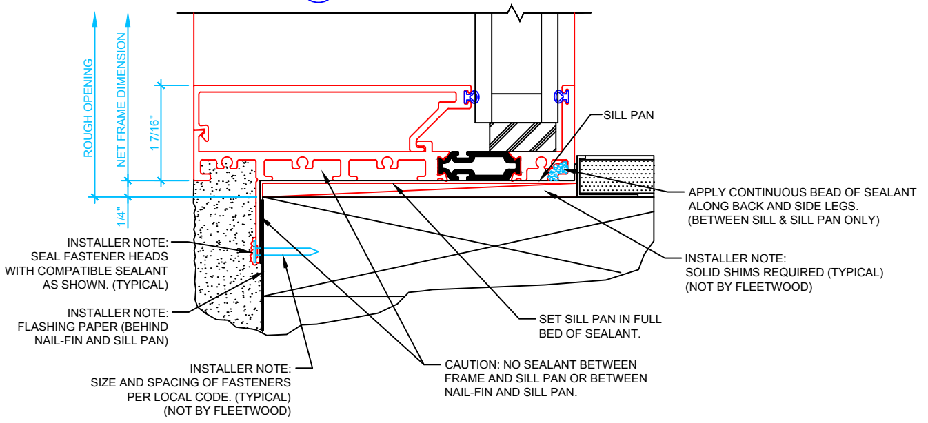
2 FIXED WINDOW SILL SCALE: 6" = 1'
