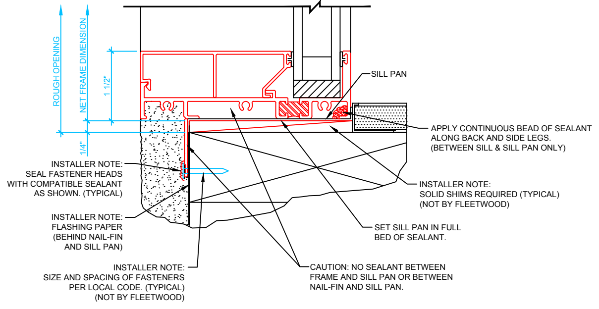
2 FIXED WINDOW SILL SCALE: 6" = 1'
