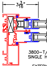
11 BLOCK JAMB
