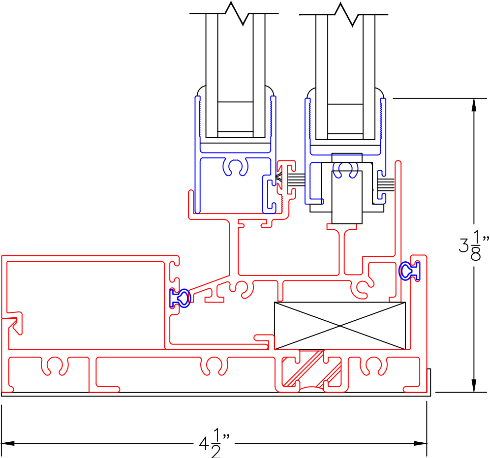
3800-T SILL WITH 250 XO SLIDER INSERT
