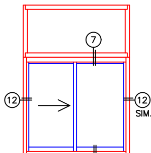
O/XO WINDOW
