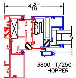
10 BLOCK JAMB
