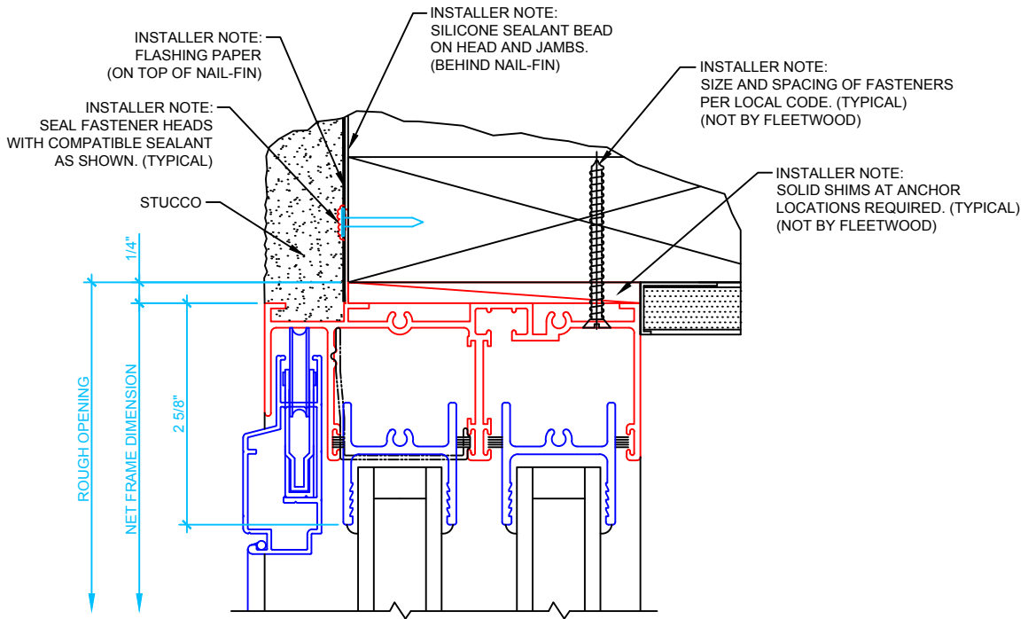
1 DOOR HEAD SCALE: 6" = 1'
