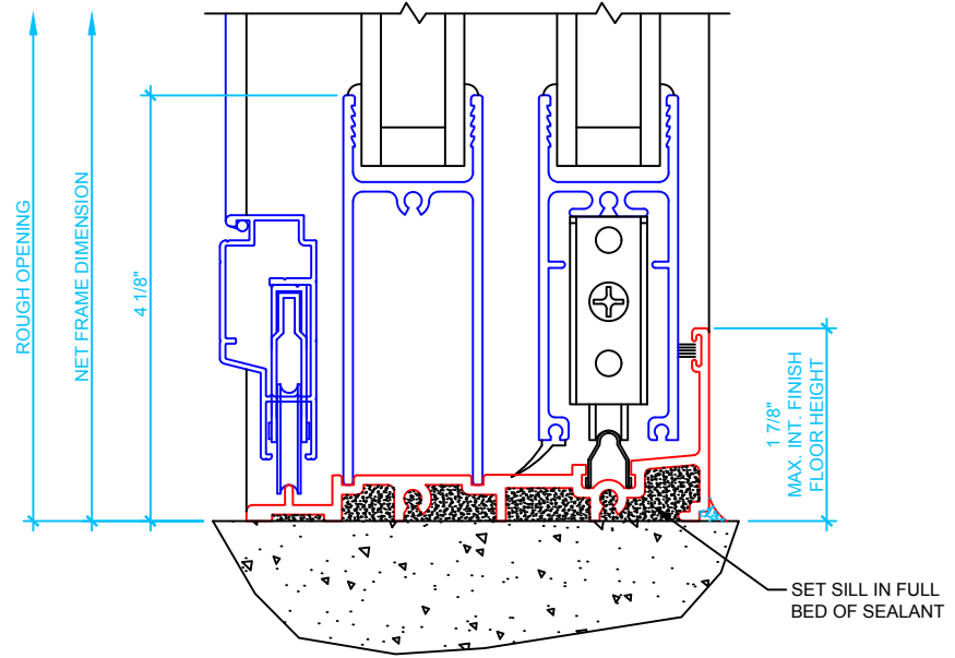
2 DOOR SILL SCALE: 6" = 1'
