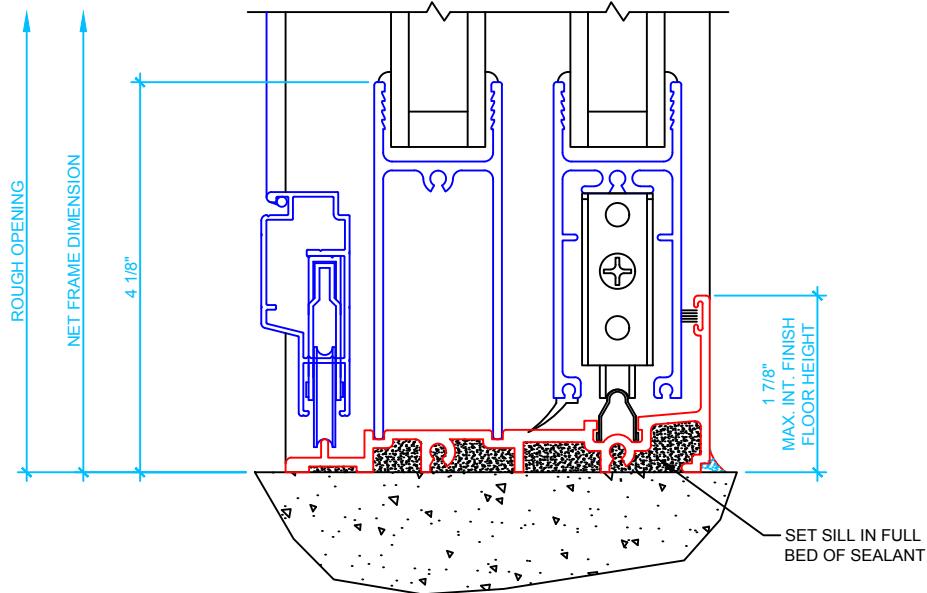
2 DOOR SILL SCALE: 6" = 1'
