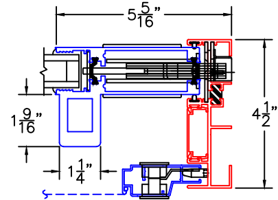
HP1-T ARCHETYPE LOCK JAMB
