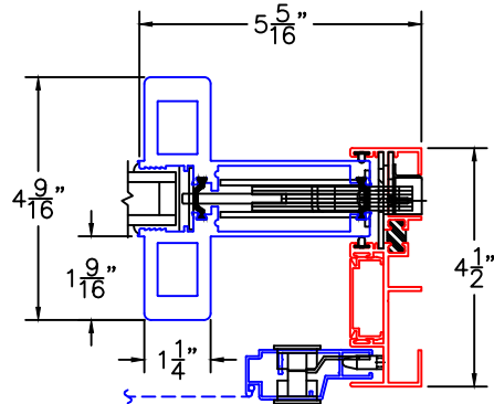
HP2-T ARCHETYPE LOCK JAMB
